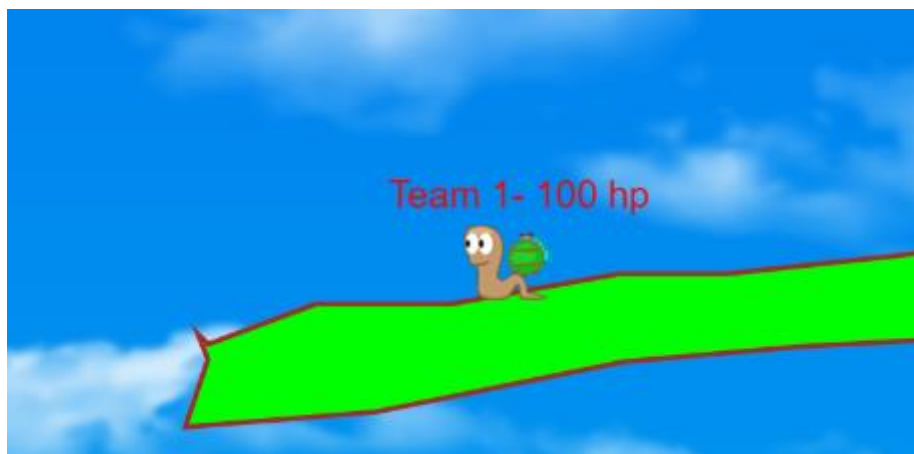
Obrázek 4 Samotný worm
